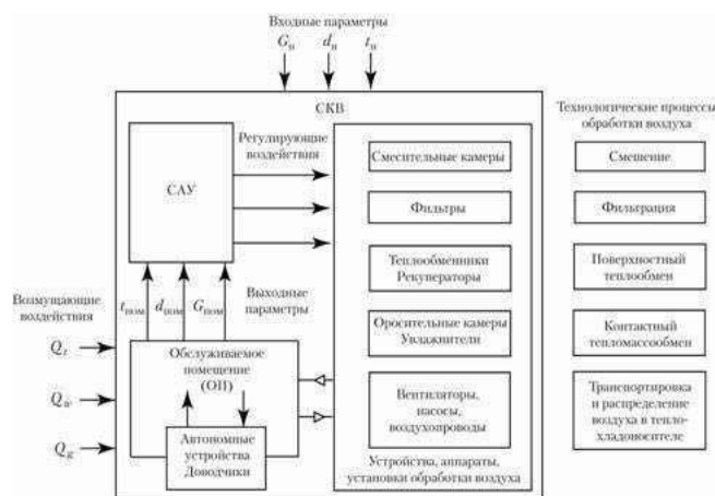
4.2 - сурет - Автоматтандыру объектісі ретінде СКР-нің жалпыланған құрылымдық сызбасы:
