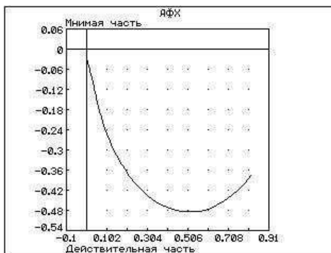
5.2 - сурет – Тұйық жүйенің амплитудалық-фазалық сипаттамасы
