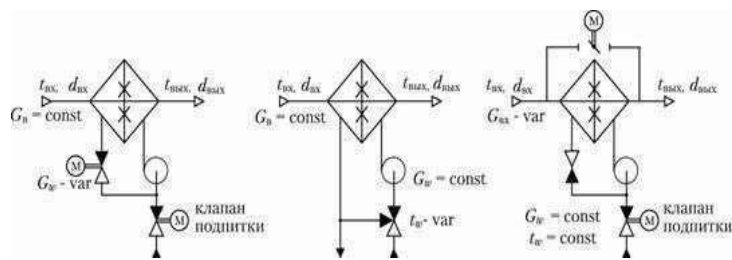
4.6 - сурет – Суару камерасын басқару әдістері:
