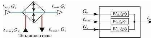
7 - сурет - «Сұйық-ауа» жылуалмастырғыштың функционалдық және құрылымдық сызбасы
