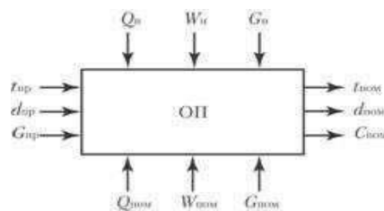
4.3 - сурет - Қызмет көрсетілетін үй-жайлардың жалпыланған функционалдық моделі (ОП) реттеу объектісі ретінде жүзеге асады
