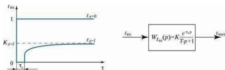
4.7 - сурет - Ауа өткізгіштің басқару объектісі ретінде сипаттамалары: а - температураның уақытша өзгеруі; б - беру функциясы.
