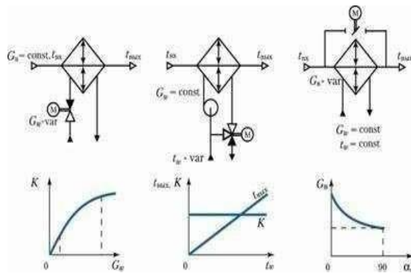
4.5 - сурет - «Сұйық-ауа» типті жер үсті жылуалмастырғыштарын басқару әдістері
