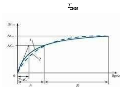
4.3 - сурет - Бөлмедегі температураны өзгерту процесі:
