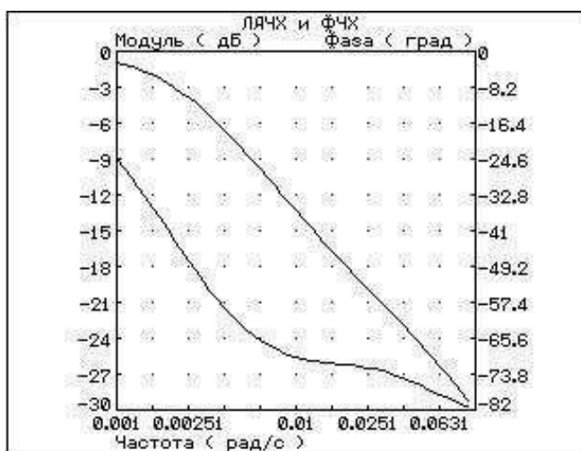
5.3 - сурет – Астатикалық реттелетін LAFC және LPFC
